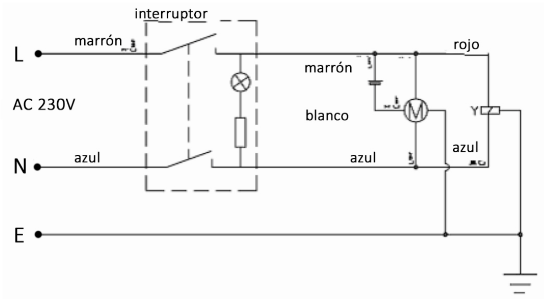
Circuito de válvula electromagnética y motor
