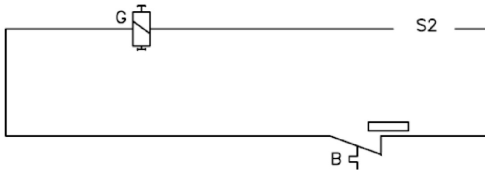
Circuito del protector de extinción de llama
